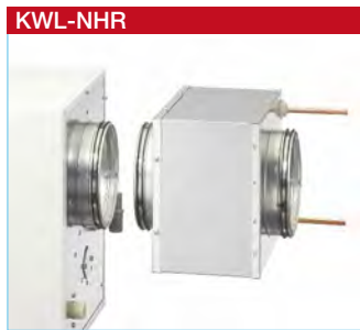
KWL-NHR Niedertemperatur-Nachheizregister (für KWL-HB.. WW)
